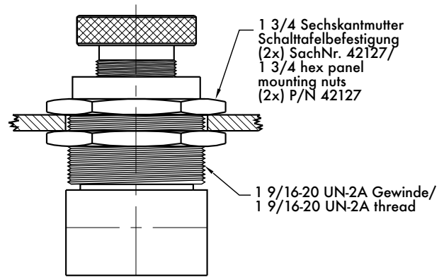
optional mit Schalttafelbefestigung/ with panel mounting optional
